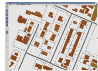
JCATS
